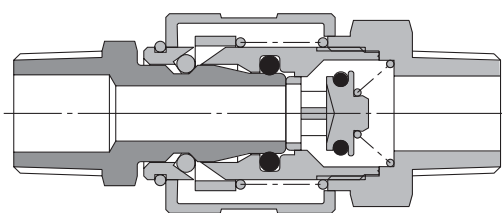
Socket
