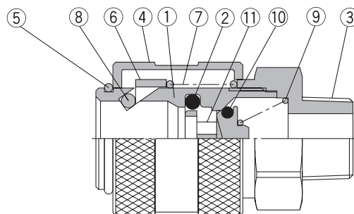
Socket
